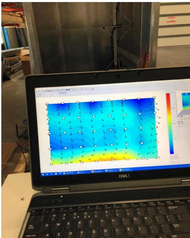
Meetresultaten luchtstromingsmetingen
